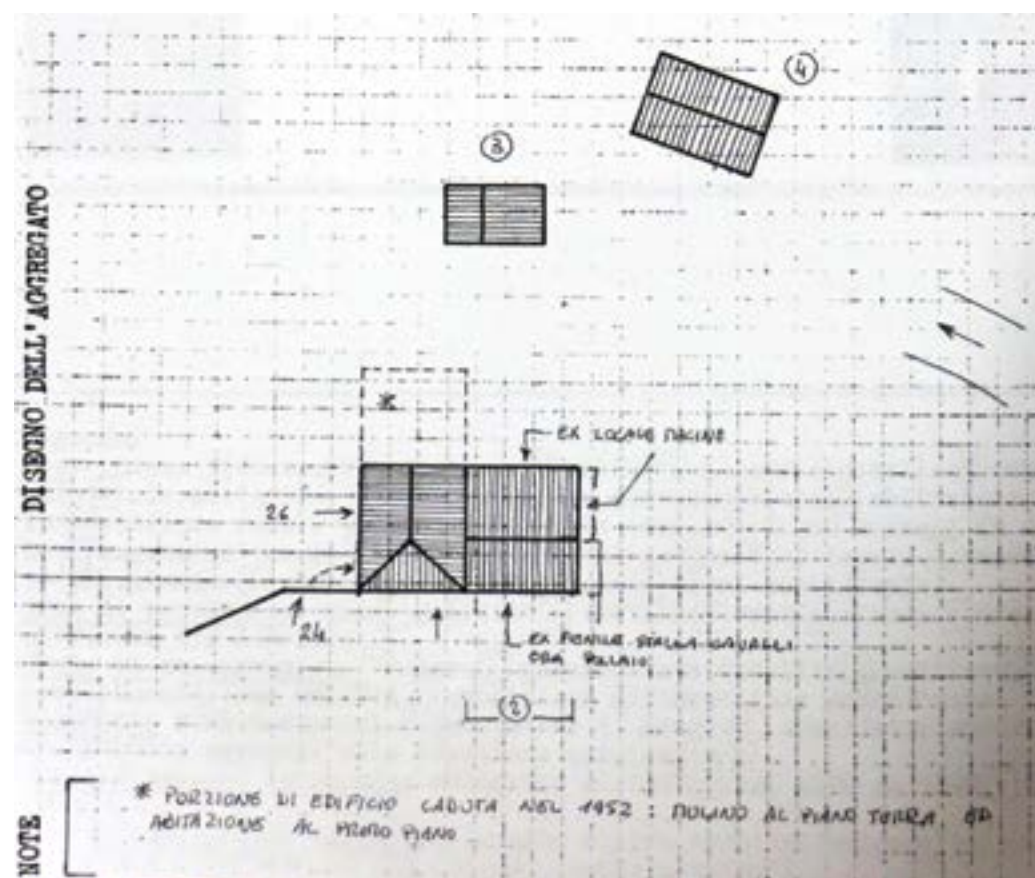
Fig. 22. Planimetria dell'aggregato edilizio del Mulino Ventura; scheda censimento patrimonio edilizio di valore storico ambientale, ottobre 1987 (Piano Regolatore Generale Comune di Sasso Marconi, Variante Generale 1990).
