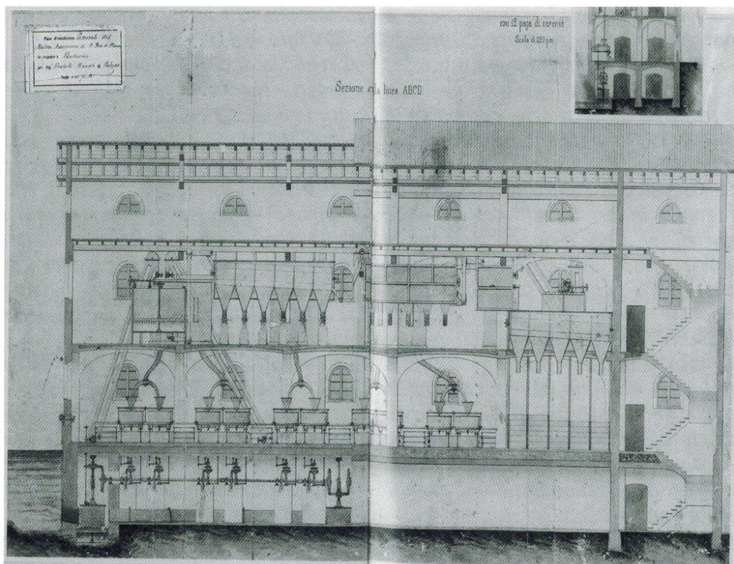
Fig. 14. Il mulino cosiddetto "all'americana" dei F.lli Monari a Pontecchio. Gli impianti erano stati installati dalla ditta Calzoni nel 1867. Disegno della sezione longitudinale dal progetto del 1867 (da "1834 1984, centocinquant'anni di vita della Calzoni", Bologna, 1984).
