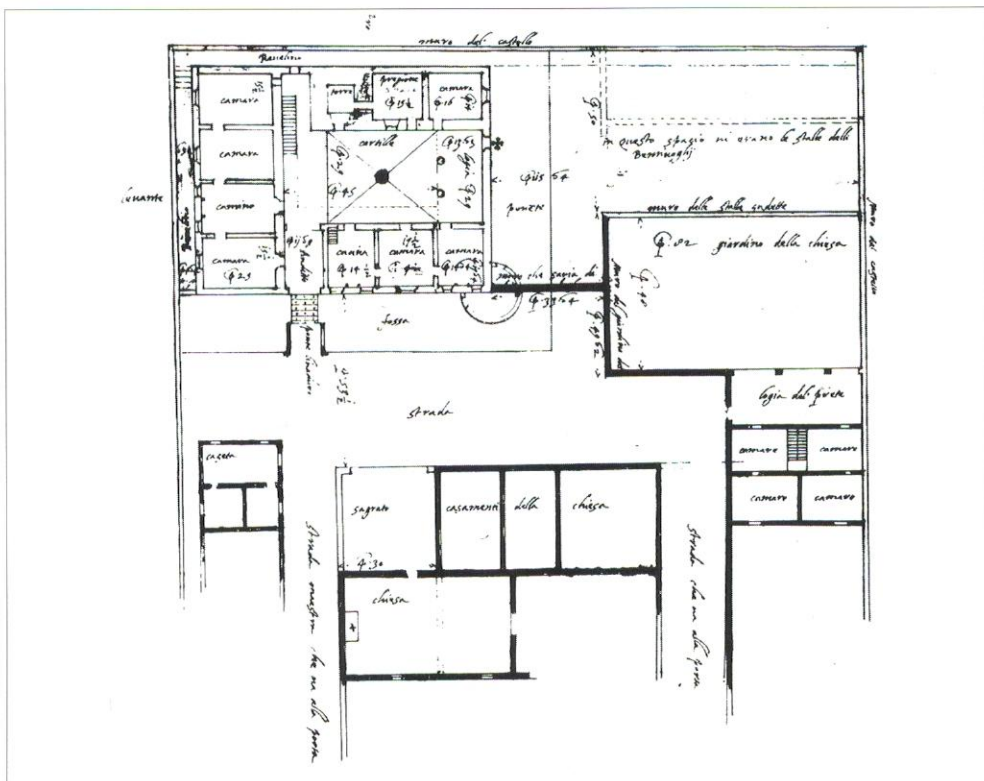
Fig. 2: Pianta del piano terreno della Rocca e della chiesa realizzata nel 1585 da Pietro Fiorini (A.S.Bo, Assunteria del Governo del Contado). La chiesa conserva ancora l'originario orientamento (tratta da Una Rocca nella storia, Catalogo della Mostra, Bologna 1989, p. 43)
